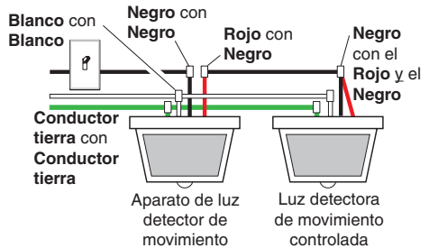
Dos lámparas detectoras de movimiento (trabajando de independientemente)
